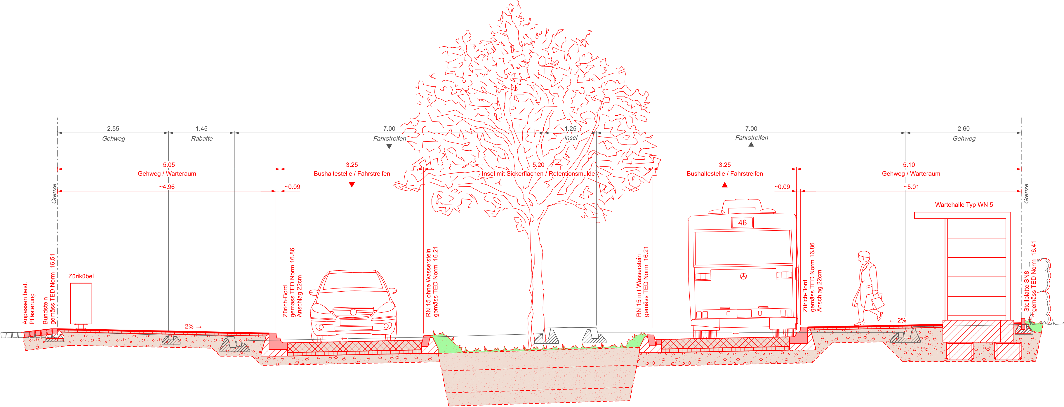
Schnitt A - A 1:50
