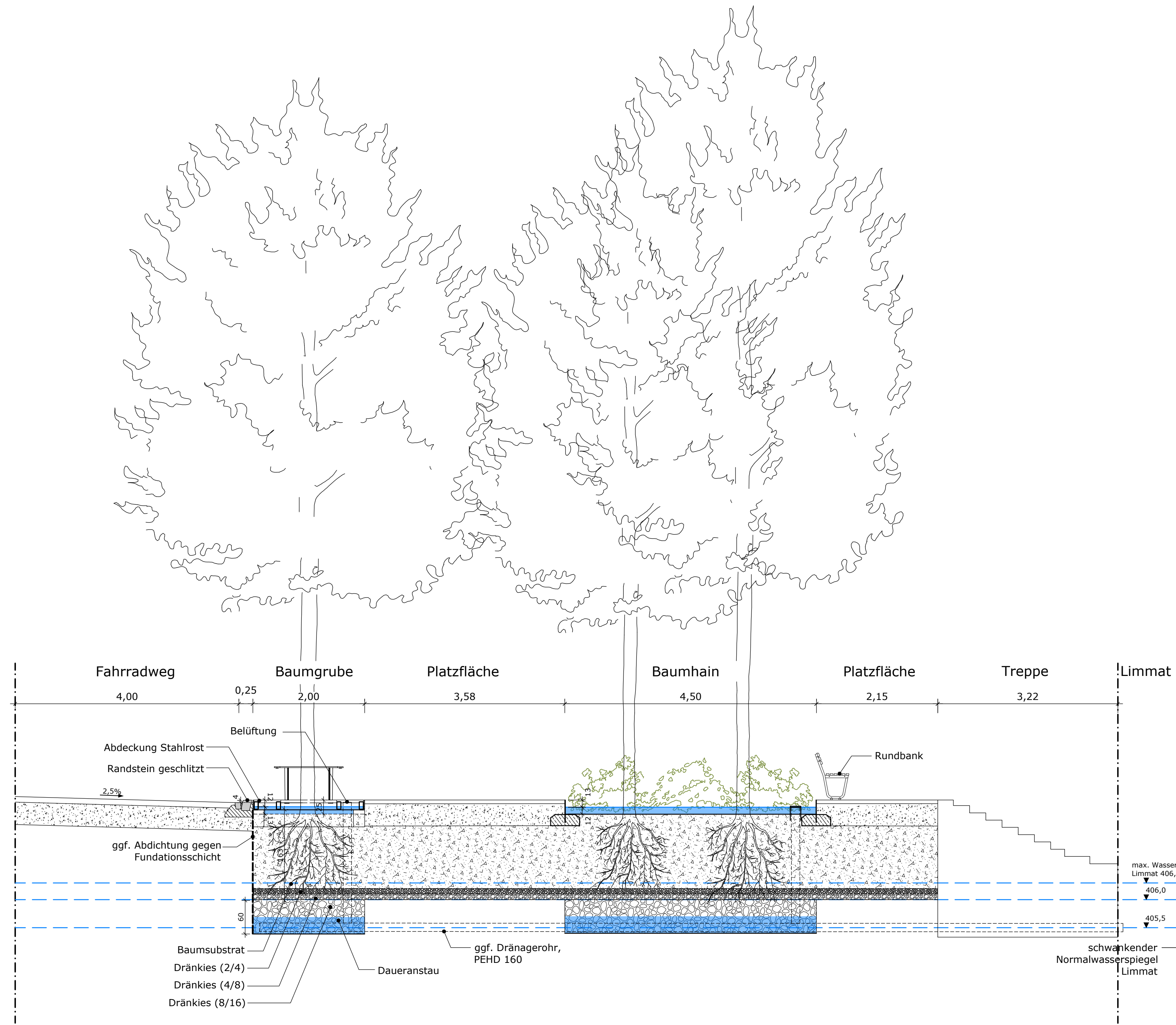
G Baumstandorte mit Baumrigole 20P02 1:50
